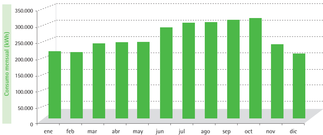
CURVA ANUAL DE DEMANDA DE ENERGÍA ELÉCTRICA Hotel Urbano *** 380 habitaciones
