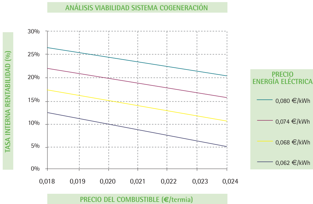
Figura 31. Análisis de sensibilidad de un proyecto de cogeneración
